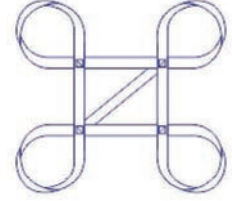
Tek çaprazlı yonca yaprağı şekilli yükleme sapanı
